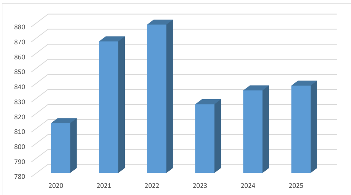
Wykres 6 Ilości odpadów (w Mg) wytworzonych w latach 2020 – 2025.
